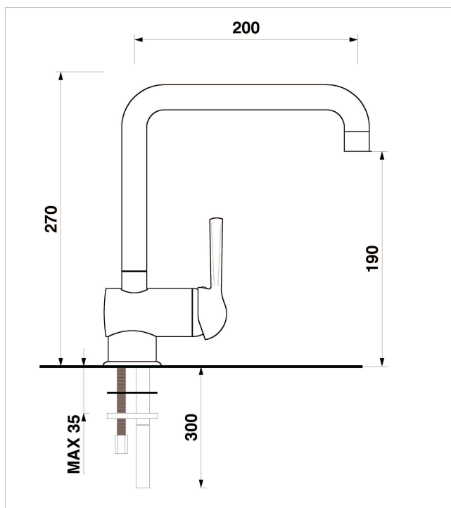
Cod. 3227 - Miscelatore canna alta quadra
